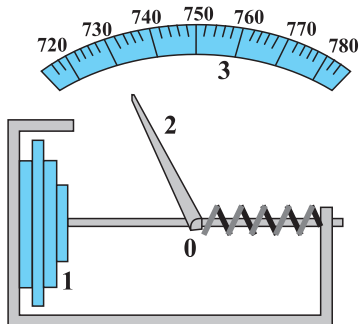
Рас. 5.46 Анероид.
